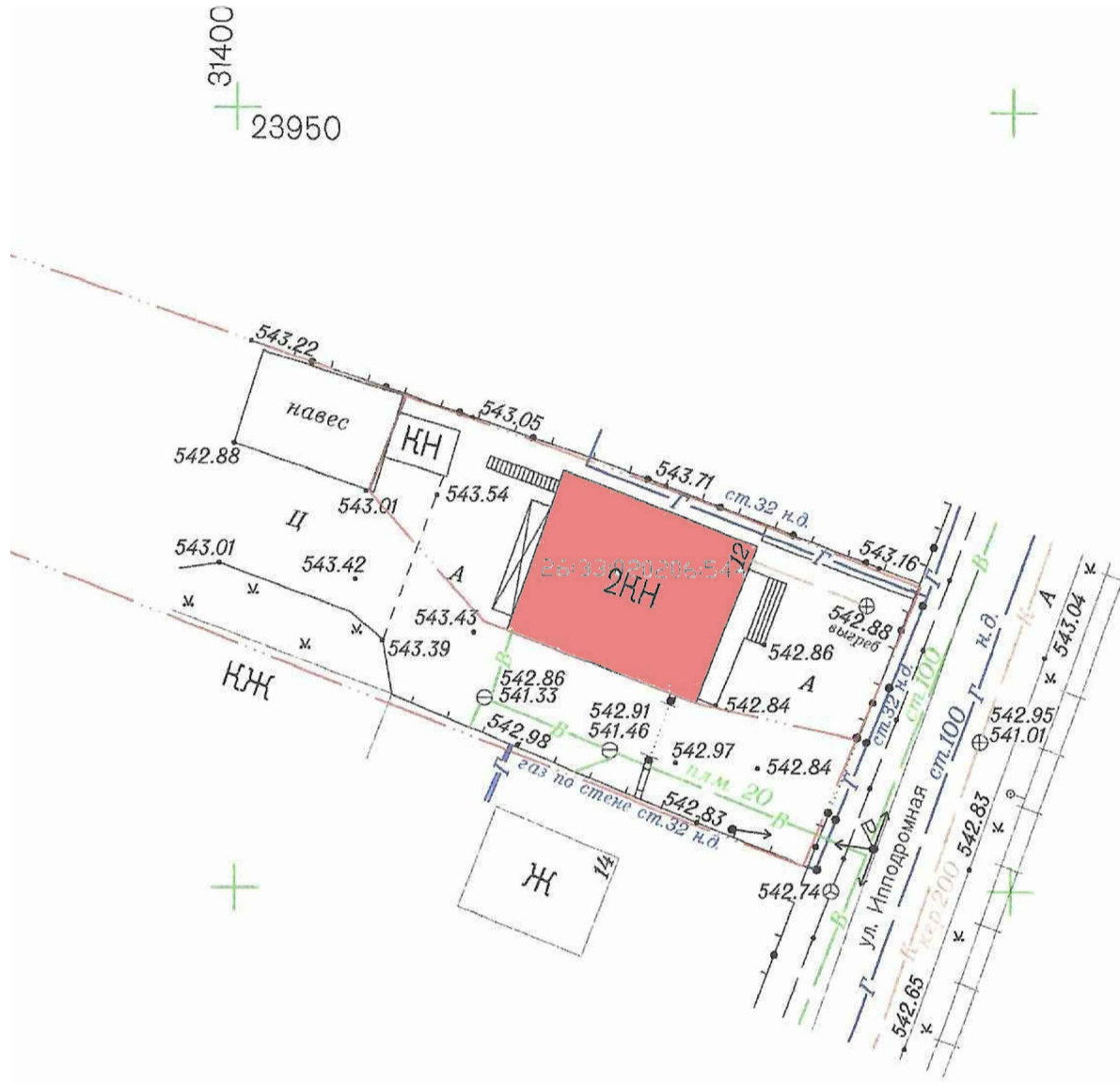
Схема генплана
