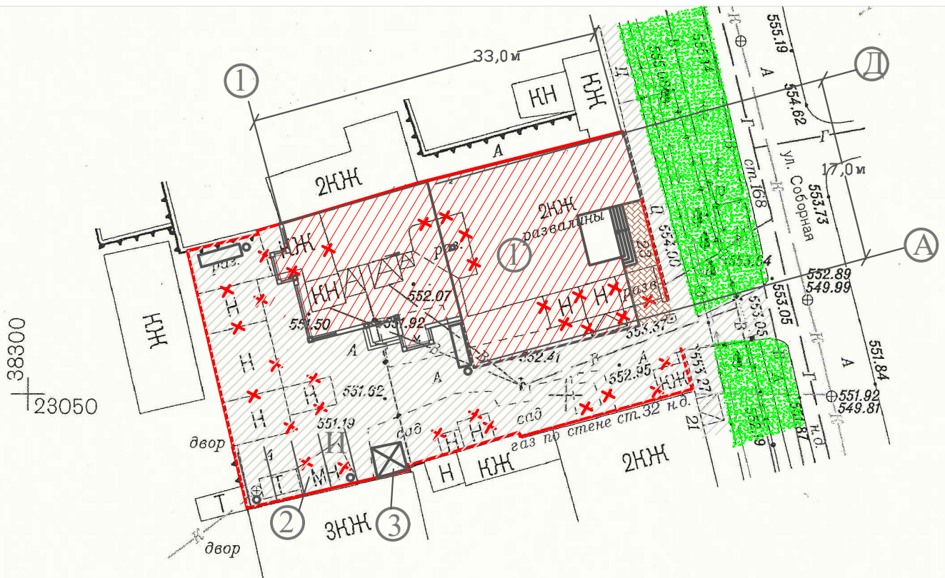
Схема генплана
